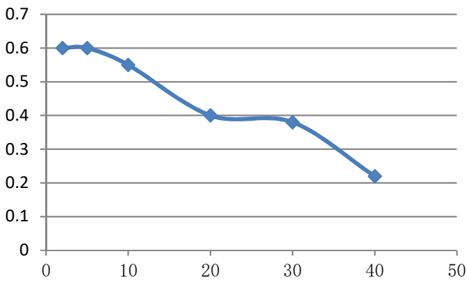
ZH30壓力與熱阻關係圖
