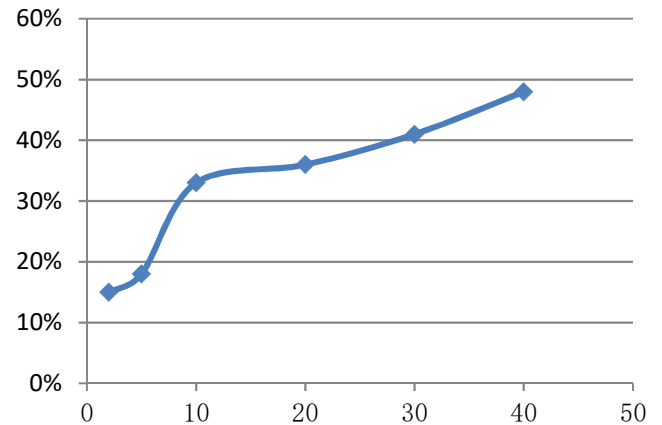
ZH30壓力與壓縮比例關係圖
